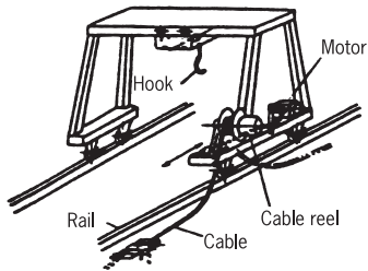
Gantry crane ※
