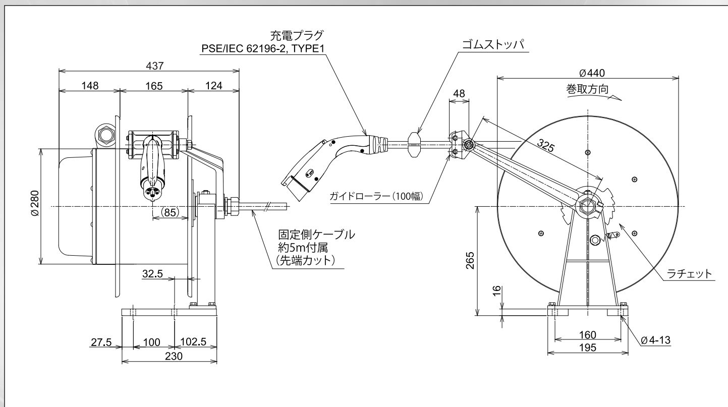
外形図
